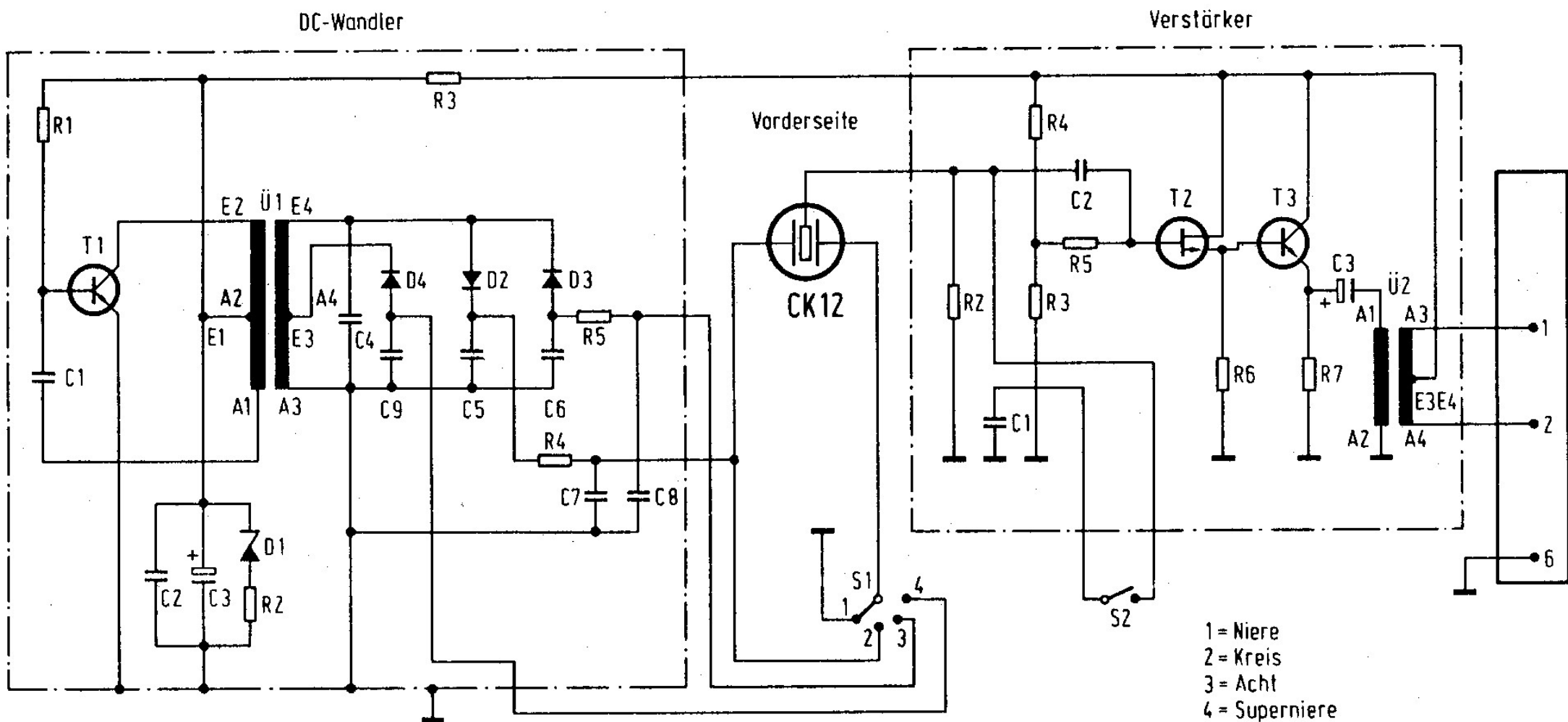
Innenschaltung des Kondensator-Mikrofons C 414 von AKG
