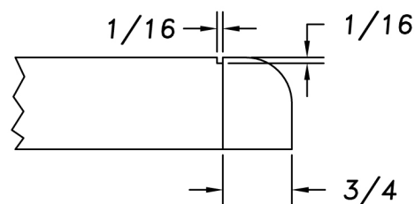
EDGE DETAIL
