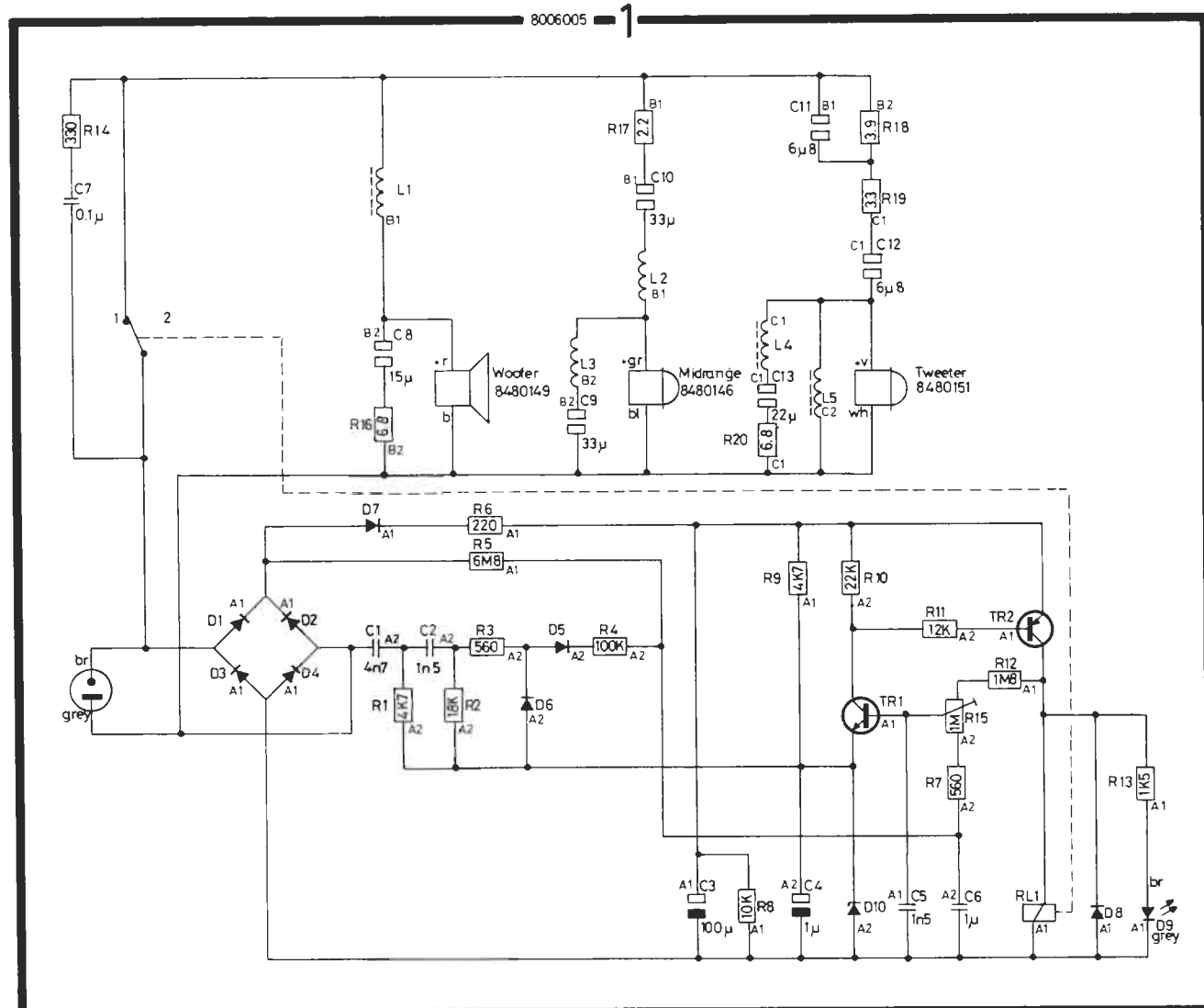
Elektrisk styklister/ List of Electrical Parts 8006005, PC1
