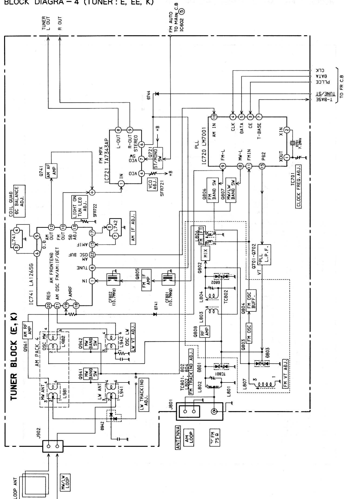
BLOCK DIAGRA - 4 (TUNER : E, EE, K)
