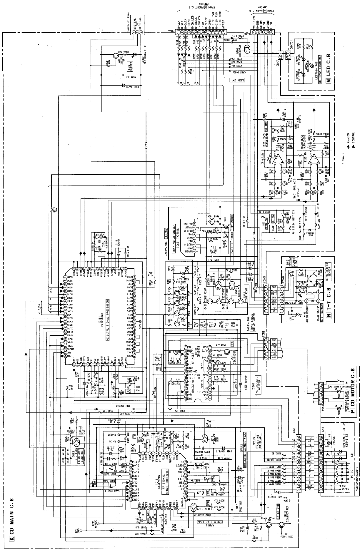
SCHEMATIC DIAGRAM - 4 (CD)
