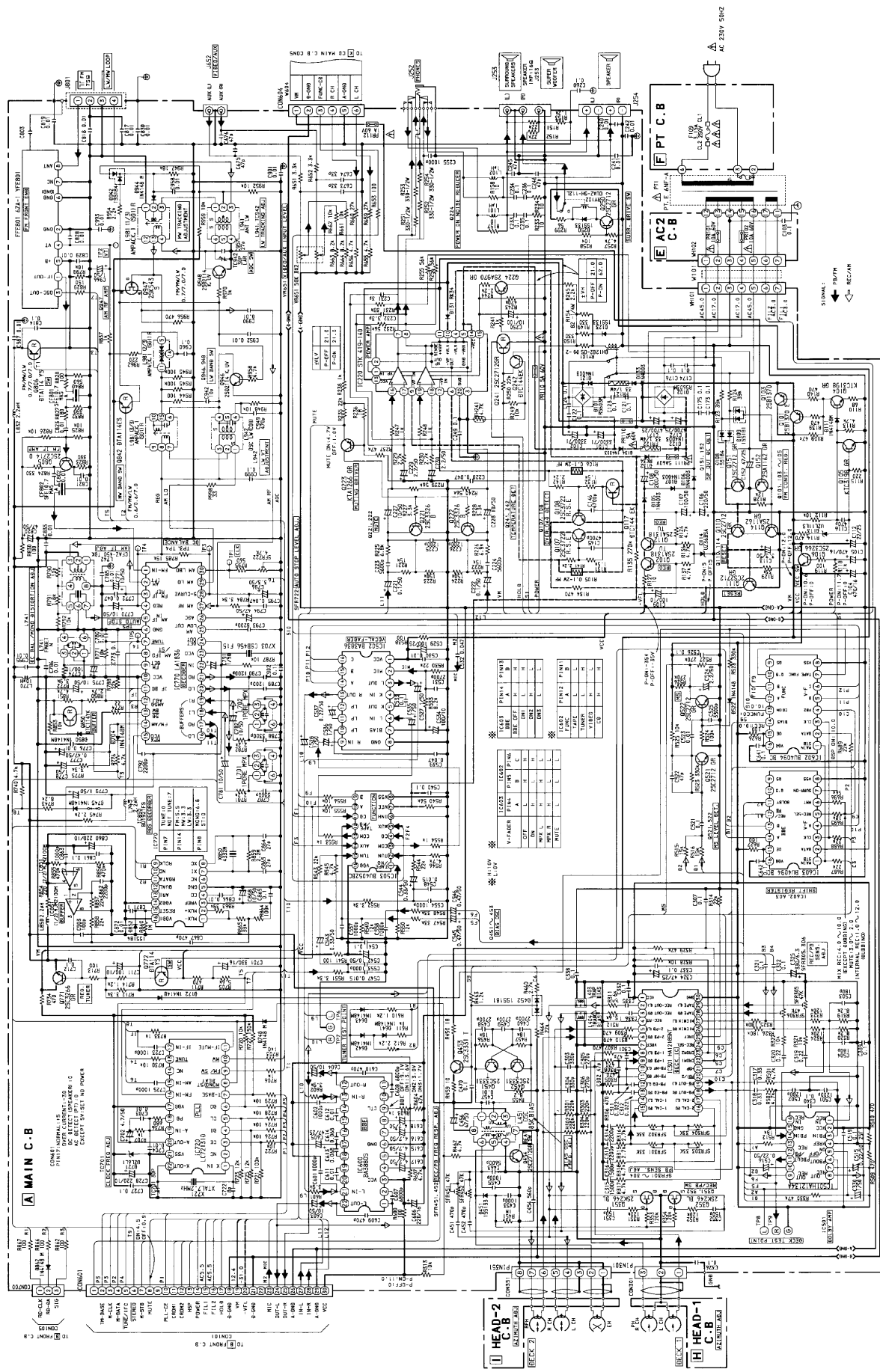
SCHEMATIC DIAGRAM - 1 (MAIN : EZ, K)
