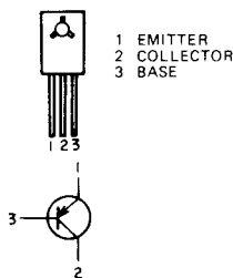
Q103: 2SA794
