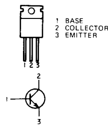
Q115: 2SD313 Q504
