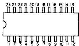
U907: TMM2016P-2
