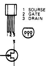
Q109: 2SK246 Q501
