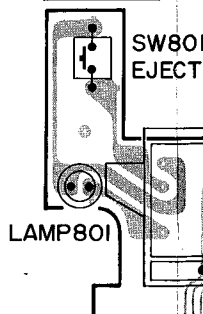
PCB-12 LCD
