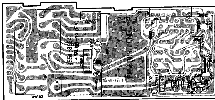
PCB-2
