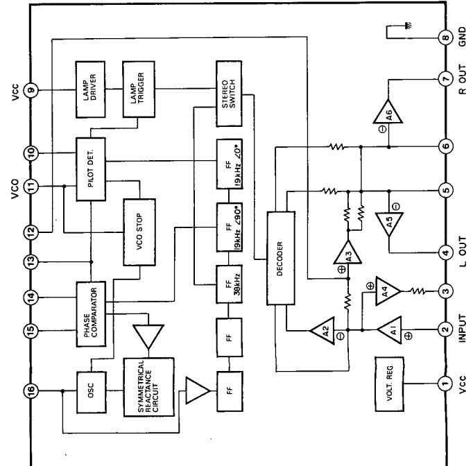
IC301 : LA3410 FM PLL MPX
