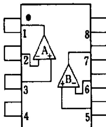
NJM2068M, pre-amp, SMD
