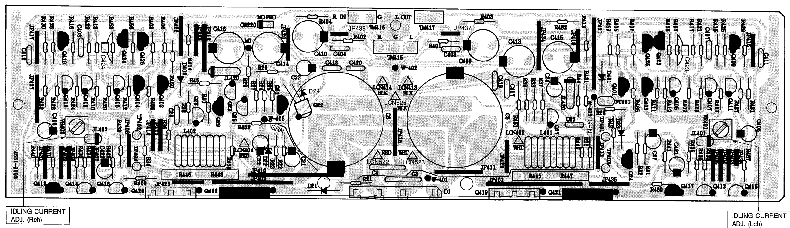
PCB-1 Main P.C.Board
