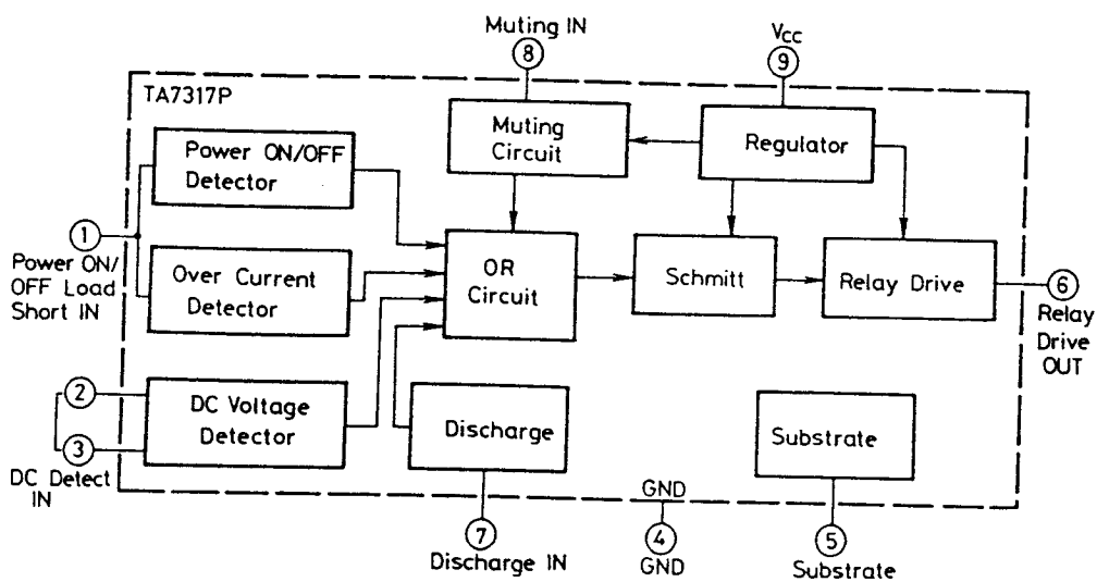
IC901: TA7317P
