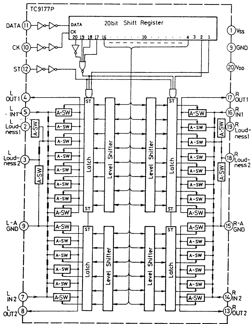
IC371: TC9177P
