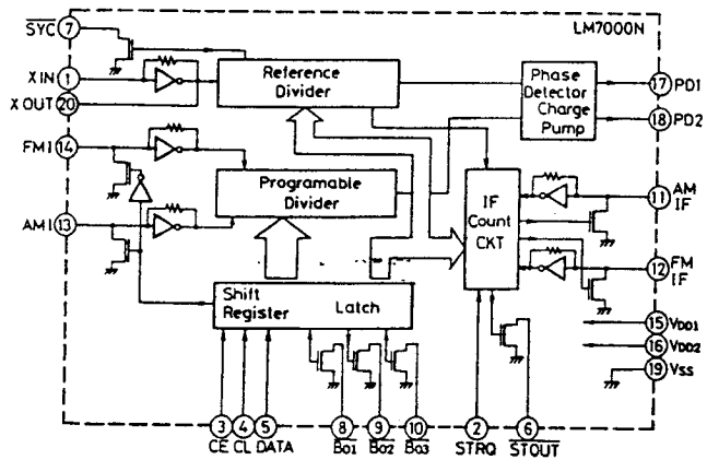
IC251: LM7000N
