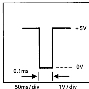
IC802 Pin2
