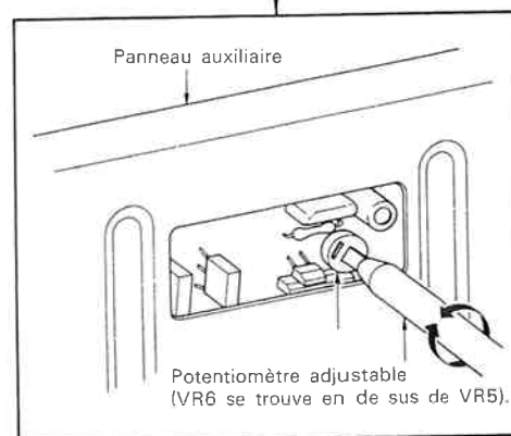
Fig. 2. Réglage de la tension de décalage (offset) en section ampli de puissance.
