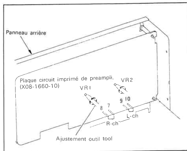
Fig. 1. Réglage de la tension de décalage (offset) en section préampli.
