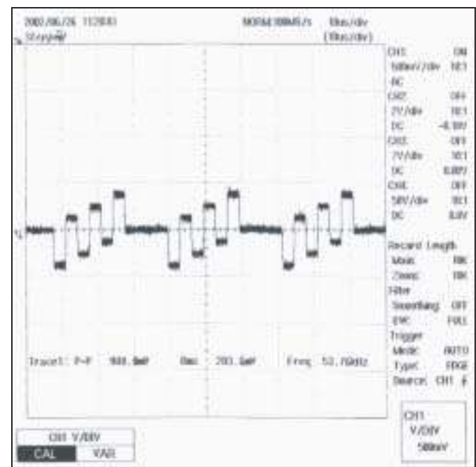
IC11 PIN 25 (DAO_B)
