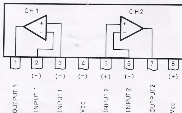
M5218L(OP Amp.)
