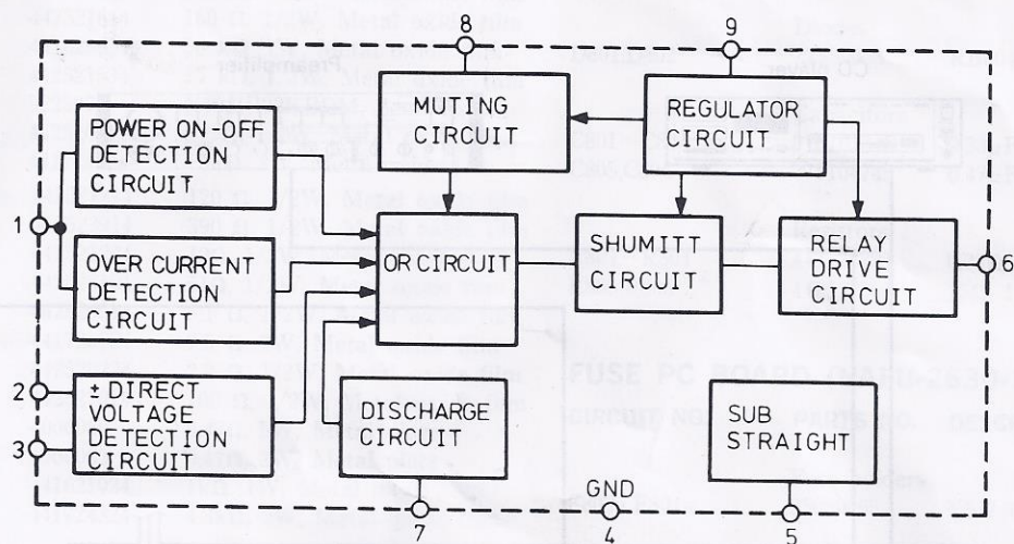
TA7318p(Meter Dirver)
