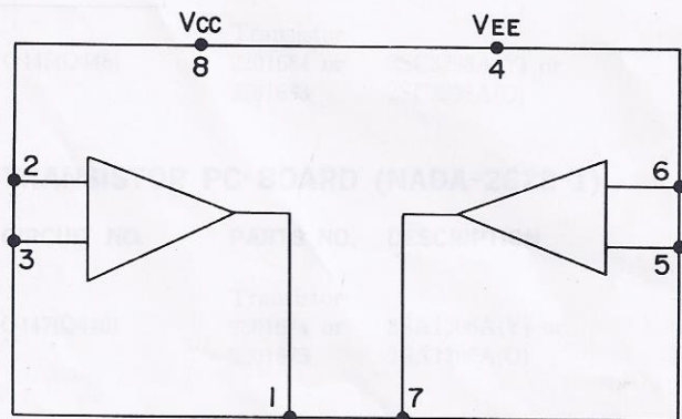
NJM4558(OP Amp.)
