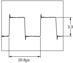
(WF04) SAI_LRCK/DIR_LRCK (SD-12:F8)
