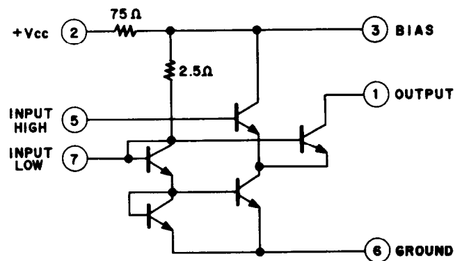
\mu PC555H (IF ampli.)
