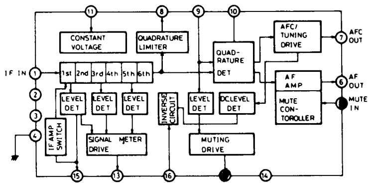
HA11225 (FM IF system)
