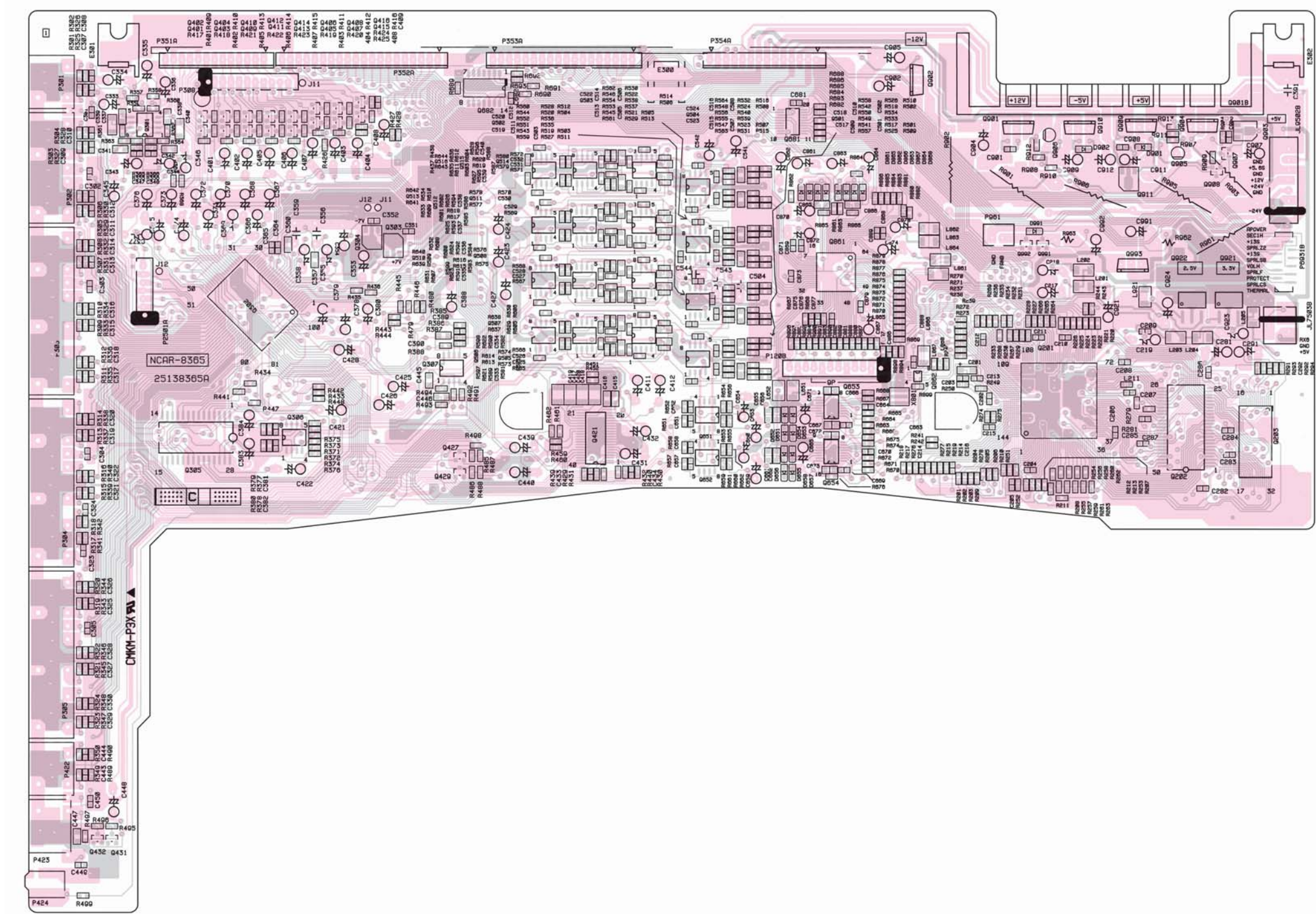
DSP and preamplifier PC board(NAAR-8365)
