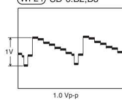
Component Y waveform (WF24) SD-6:B2,B3
