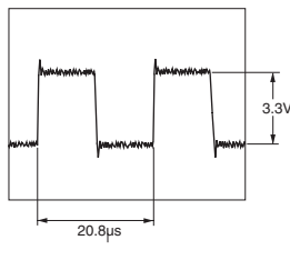
(WF07) CX_LRCK (SD-9:D4)
