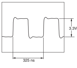
(WF08) CX_SCLK (SD-9:D4)
