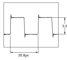
(WF04) SAI_LRCK (SD-9:B4)
