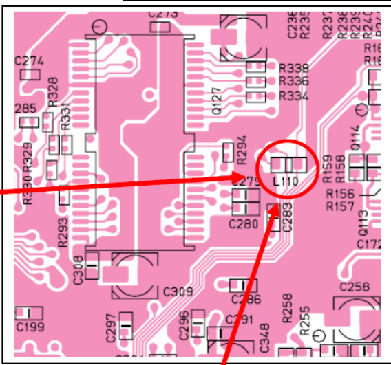
PV16-SERVO PWB
