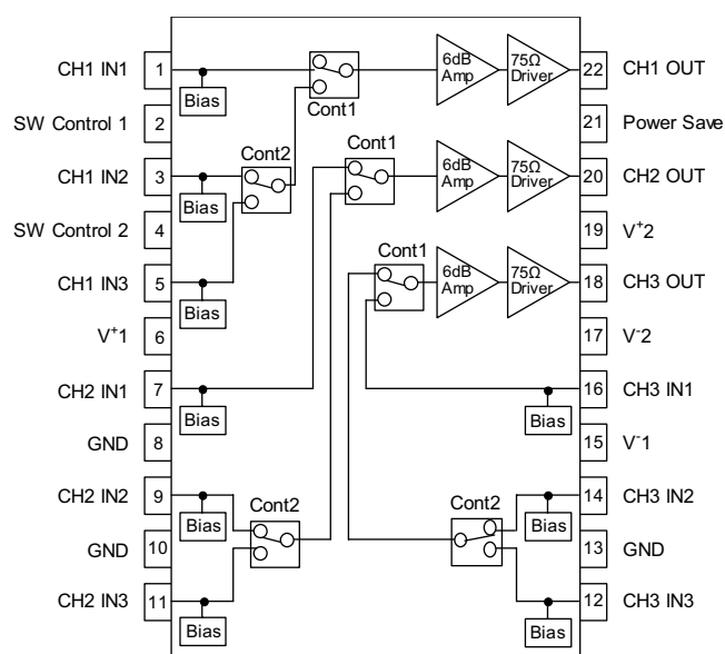
SDIP22
