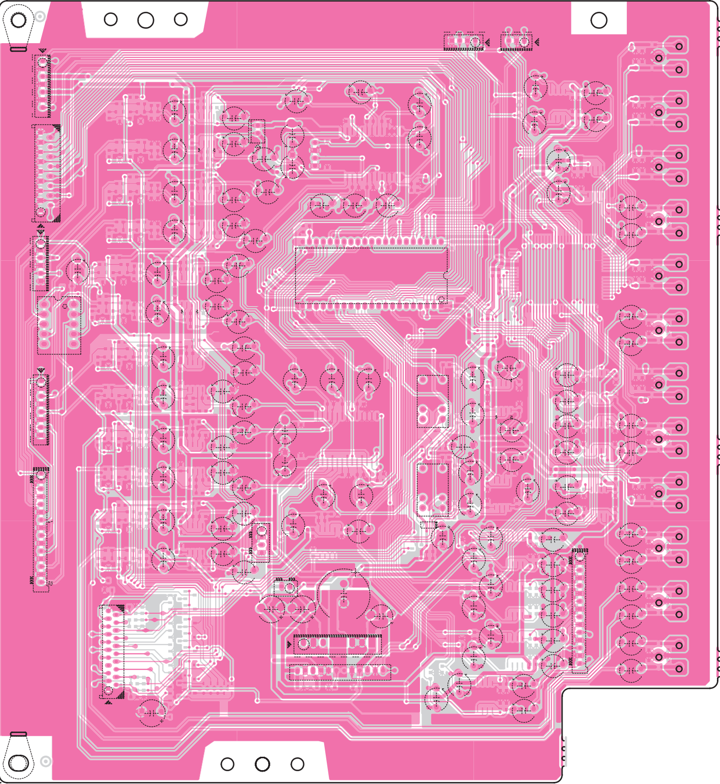
INPUT PWB B
