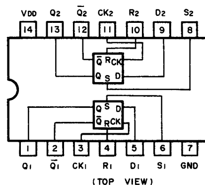
Fig. 13.13 D-Type Flip-Flop C-MOS IC TC4013BP
