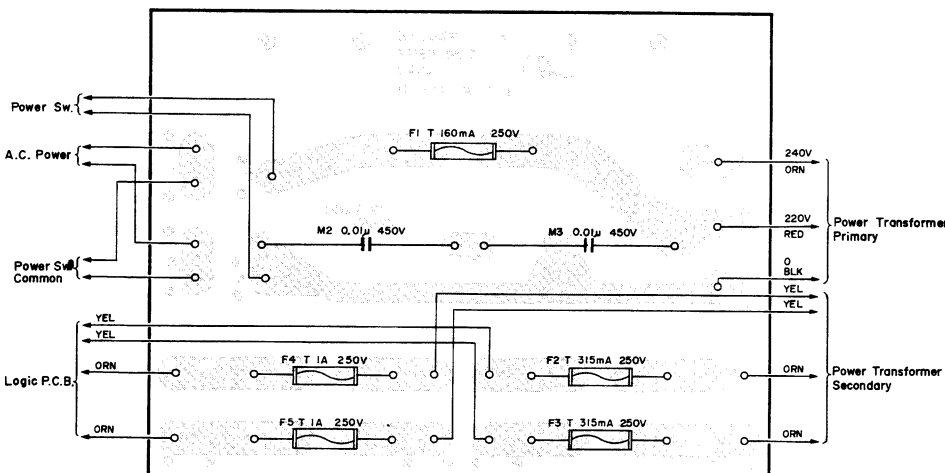
Fig. 7.6.4 220 V Class 2
