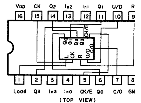
Fig. 13.14 BCD Up/Down Counter C-MOS IC
