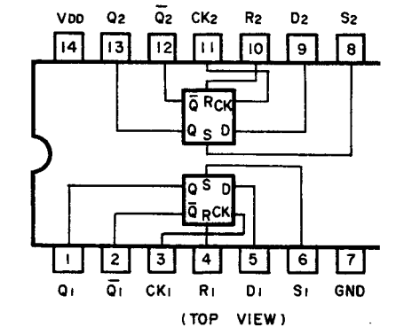
Fig. 13.13 D-Type Flip-Flop C-MOS IC TC
