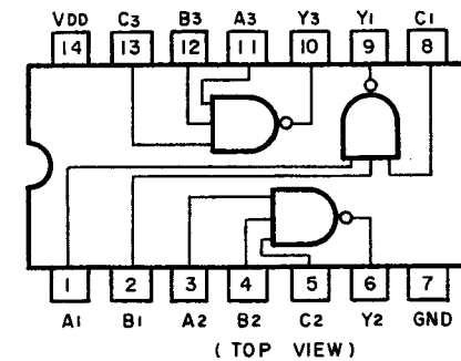
Fig. 13.9 NAND Gate C-MOS IC \mu PD4023C
