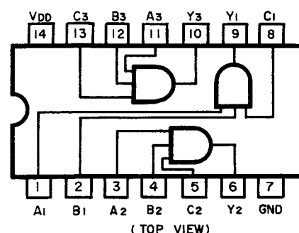
Fig. 13.12 AND Gate C-MOS IC μPD4073C
