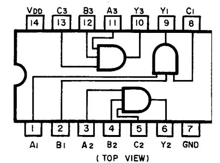
Fig. 13.12 AND Gate C-MOS IC \mu PD4073
