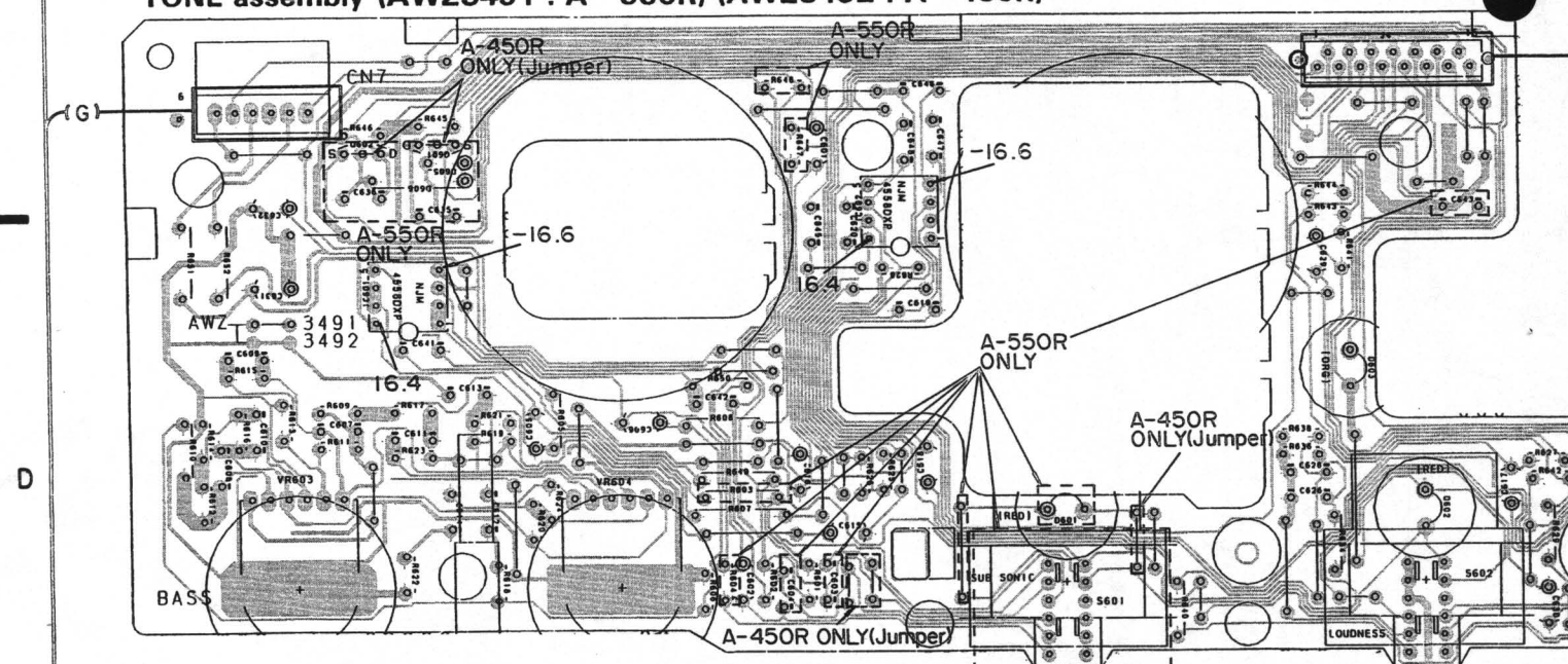
TONE assembly (AWZ3491 : A - 550R) (AWZ3492 : A - 450R)
