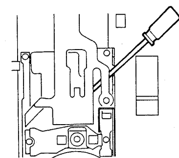
(Vue du haut) Sens d'insertion du tournevis
