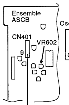
(Vue du haut) Sens d'insertion du tournevis
