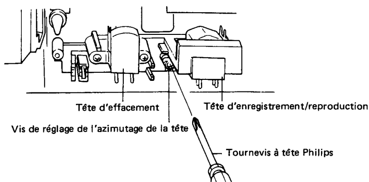
Fig. 10-3 Réglage de l'azimut de la tête
