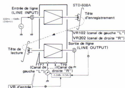
Fig. 13-9 Réglage du niveau d'enregistrement
