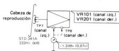
Fig. 13-6 Ajuste del nivel de reproducción
