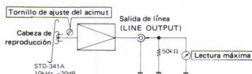
Fig. 13-4 Ajuste de acimut de la cabeza
