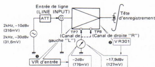
Fig. 13-3 Réglage du circuit Dolby NR
