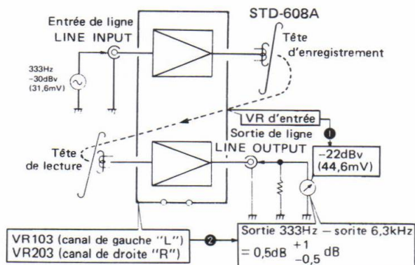
Fig. 13-8 Réglage de la réponse en fréquence enregistrement/lecture
