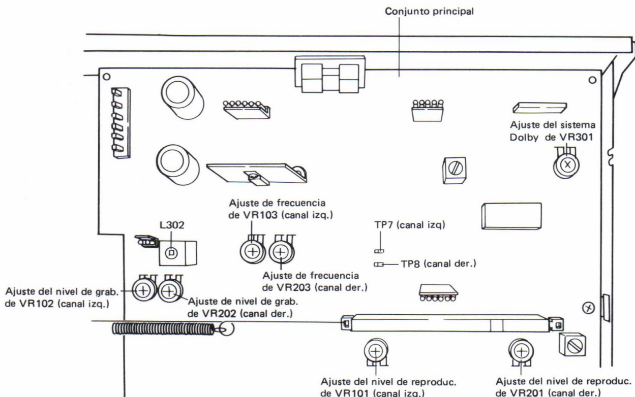
Fig. 13-2 Puntos de ajuste
