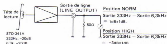
Fig. 13-5 Contrôle de l'égalisation de lecture
