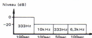
Fig. 13-1 Contenu de la bande d'essai STD-341A
