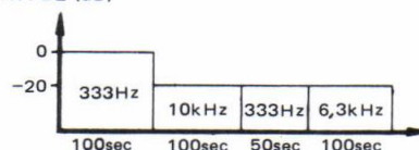
Fig. 13-1 Contenido de la cinta de prueba STD-341A
