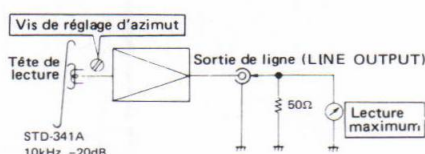
Fig. 13-4 Réglage d'azimut de la tête
