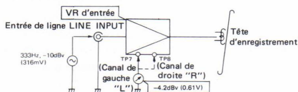
Fig. 13-7 Contrôle de l'indicateur de niveau
