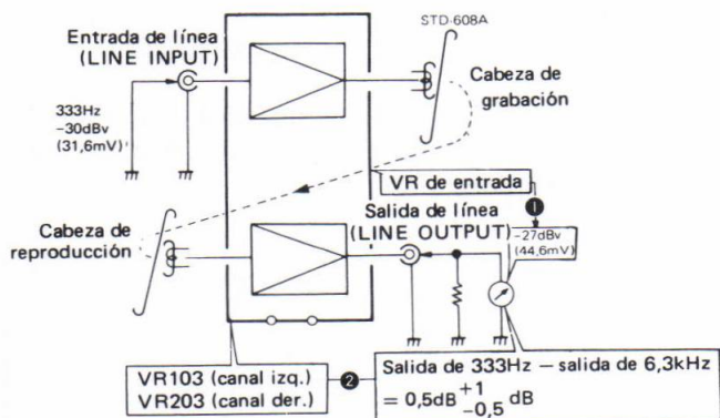
Fig. 13-8 Ajuste grabación/reproducción de la respuesta en frecuencia
