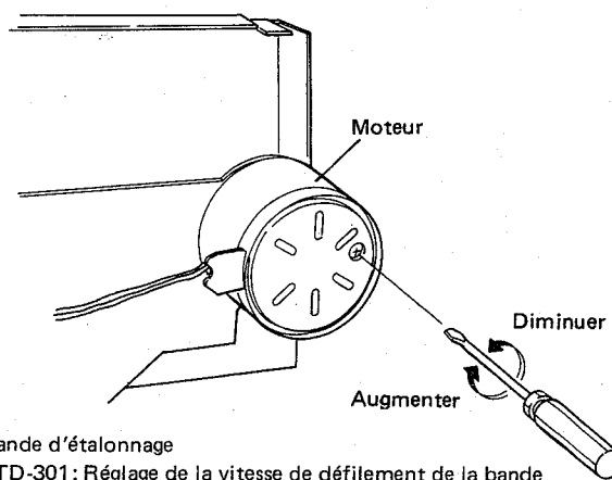
Fig. 10-2 Réglage de la vitesse de défilement de la bande
