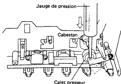
Fig. 10-1 Réglage de la force d'appui du galet-presseur
