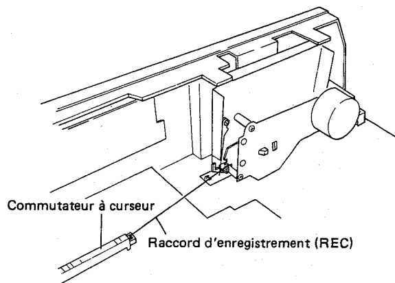
Fig. 10-3 Réglage et vérification du raccord d'enregistrement (REC)
