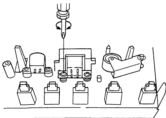
Fig. 10-5 Ajuste azimutal de la cabeza de grabación
