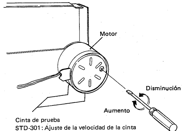
Fig. 10-2 Ajuste de la velocidad de la cinta
