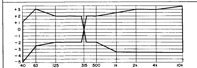
Fig. 11-10 Zona de respuesta en frecuencia permisible para grabación/reproducción (NORM)
