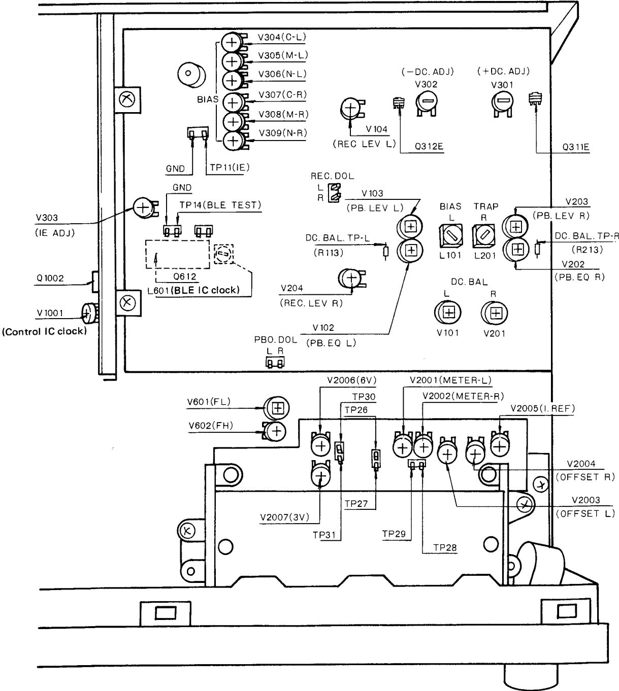
Fig. 11-6 Lugares de ajuste
