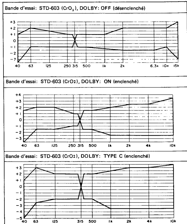
Fig. 11-12 Zone admissible de réponse en fréquence d'enregistrement/reproduction (CrO 2 )
