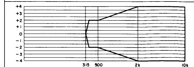
Fig. 11-13 Zona de respuesta en frecuencia permisible para grabación/reproducción (NORM, AUTO-BLE)
