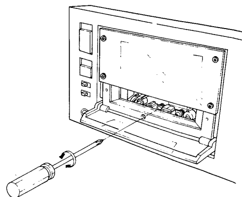
Fig. 11-8 Ajuste del acimut de la cabeza
