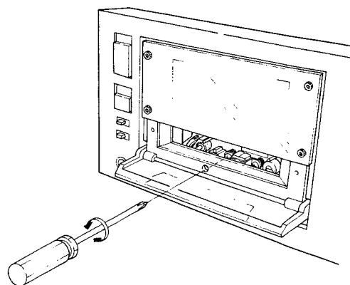
Fig. 11-8 Réglage de l'azimutage de la tête
