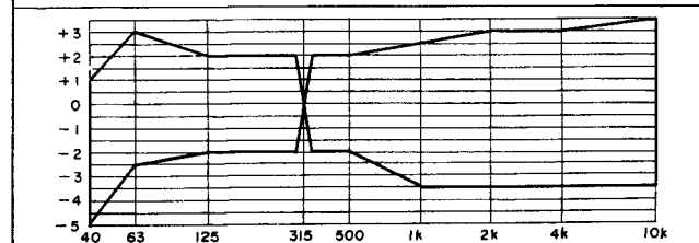
Fig. 11-11 Zona de respuesta en frecuencia permisible para grabación/reproducción (METAL)
