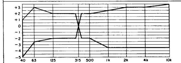
Fig. 11-12 Zona de respuesta en frecuencia permisible para grabación/reproducción (CrO 2 )
