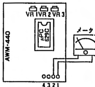
図7-3 メータアンプAss'yの調整
