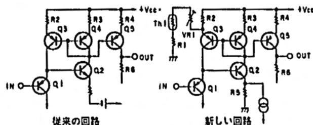
図5-2 基本回路図
