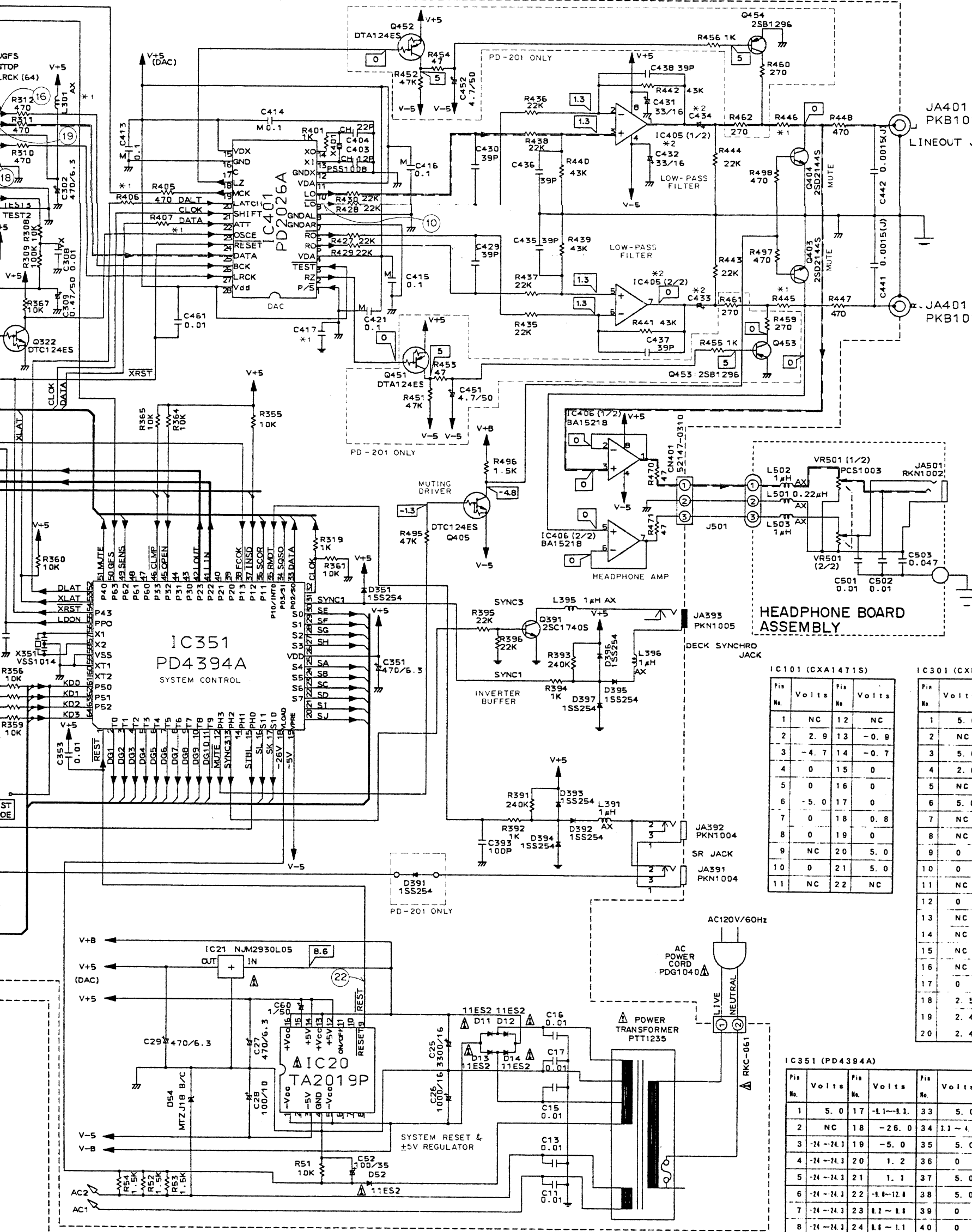
IC401 (PD2026A)
