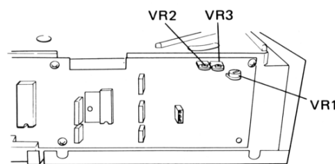
Fig. 9-3 Réglage 2 du détecteur de fin
