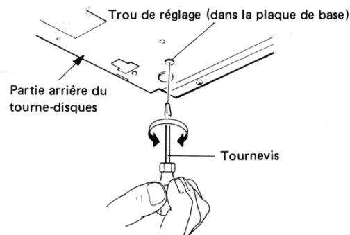
Fig. 9-1 Réglage d'abaissement de position de l'aiguille
