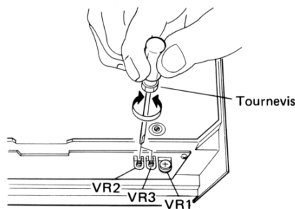
Fig. 9-4 Réglage de position
