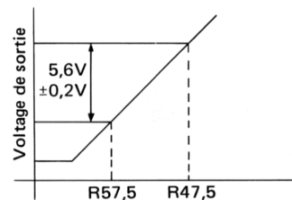
Fig. 9-3 Réglage 2 du détecteur de fin
