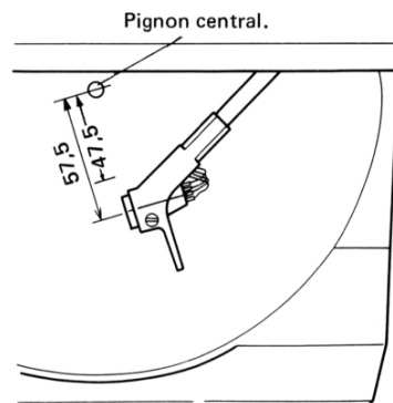
Fig. 9-2 Réglage 1 du détecteur de fin
