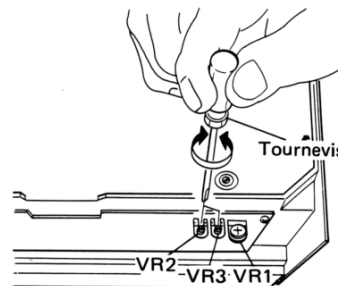
Fig. 9-5 Réglage de la vitesse du moteur phono
