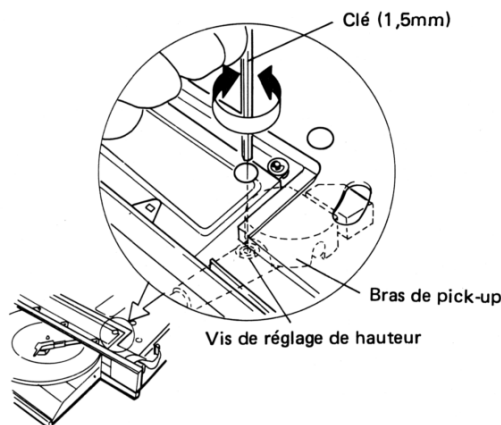
Fig. 9-6 Réglage de hauteur de l'aiguille
