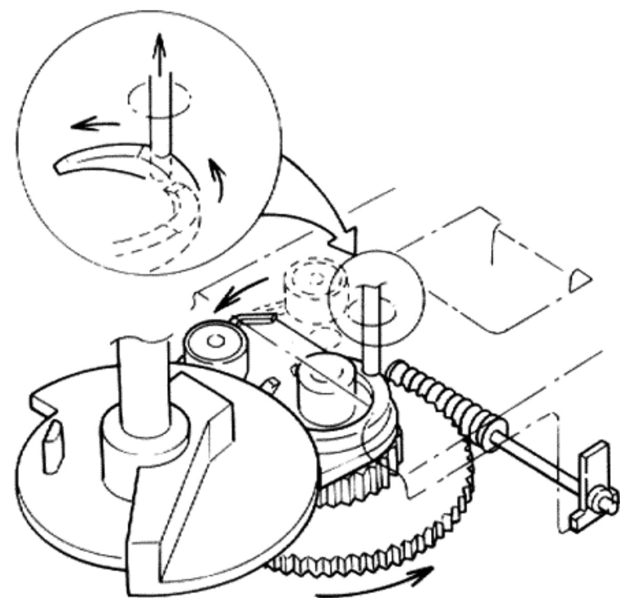
Fig. 8 Elevation down
