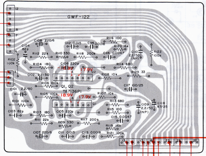
EQ Ass'y GWF-122
