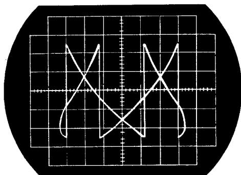
Fig. 8 Lissajous figure
