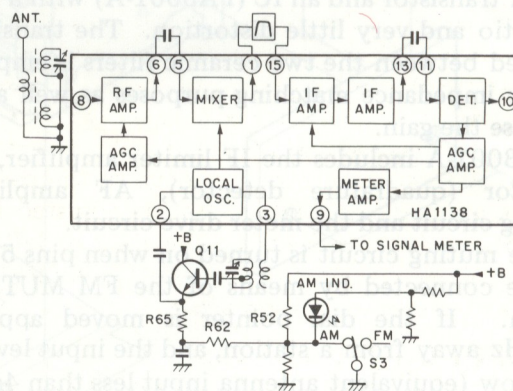
Fig. 4-1 AM tuner
