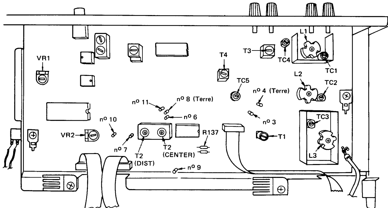
Fig. 11-1 Points de réglage et points de mesure
