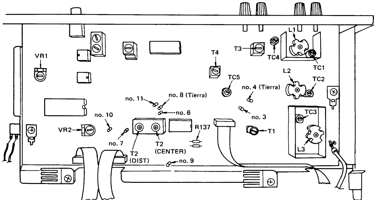
Fig. 11-1 Puntos de ajuste y puntos de medida
