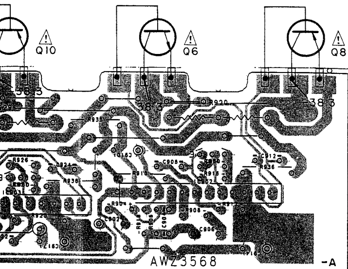
R. C. AMP assembly (AWZ3568)
