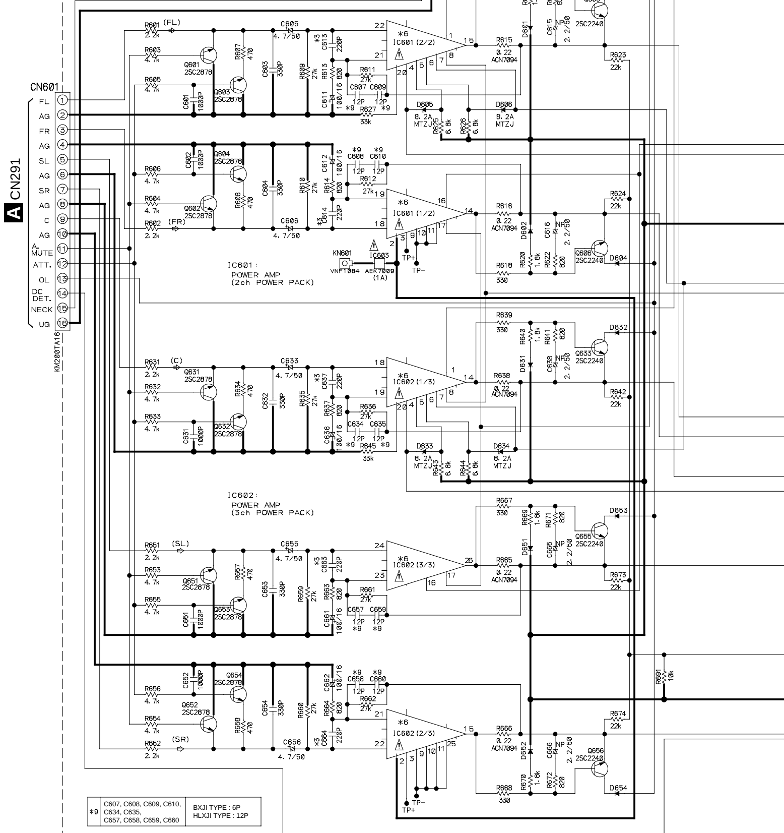
C 1/2 AMP&PRIMARY ASSY (BXJI : AWX7473) (HLXJI : AWX7388)
