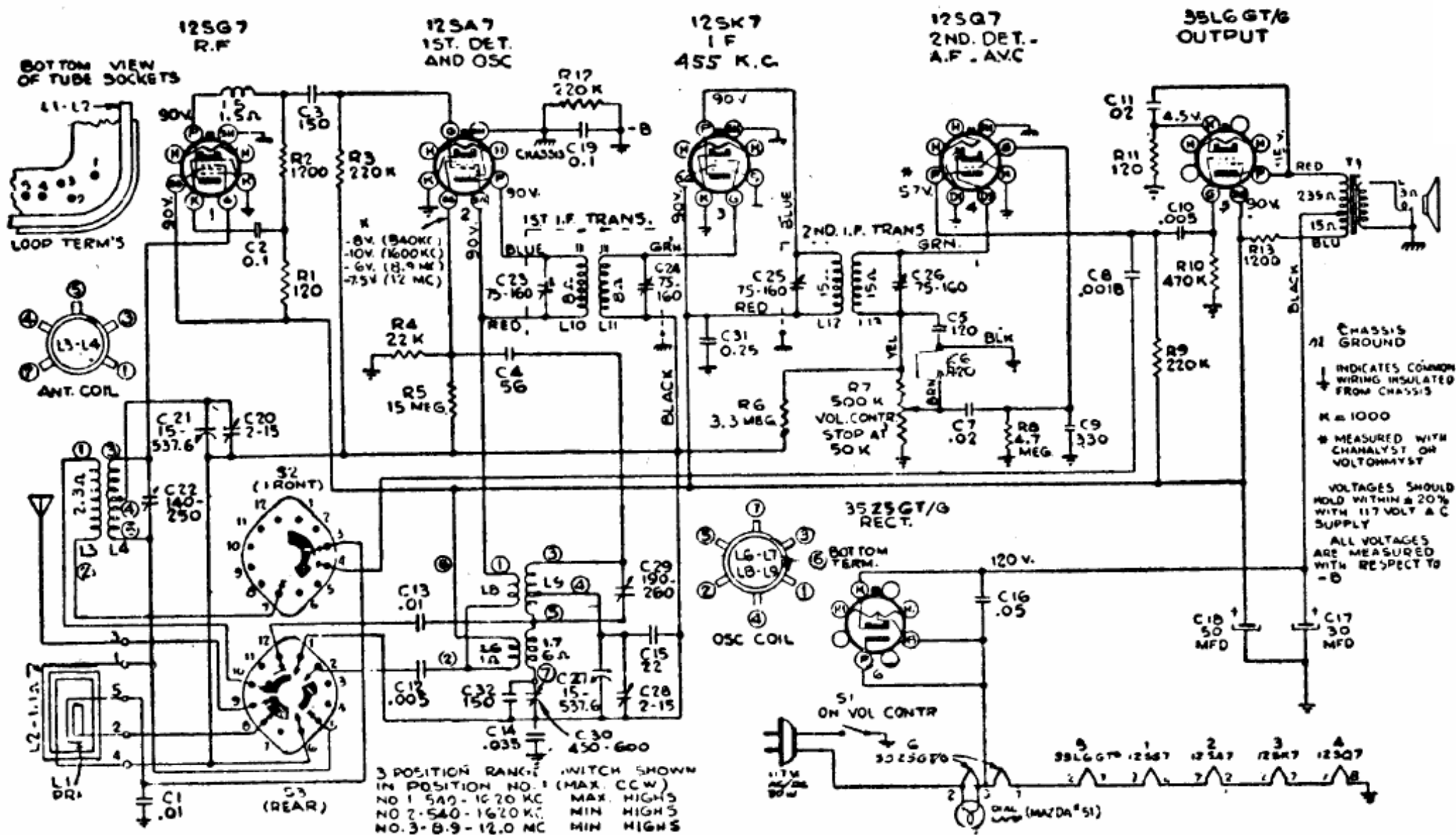
Supereterodina RCA mod. 56 X10.
