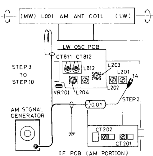
Fig. 6-b. AM (MW and LW) Alignment (RT-1000L and RX-1000L) Abb. 6-b. AM (MW und LW)-Abgleich (RT-1000L und RX-1000L) Fig. 6-b. Aligment AM (MW et LW) (RT-1000L et RX-1000L)
