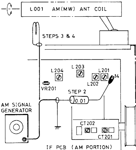
Fig. 6-a. AM Alignment (RT-1000 and RX-1000) Abb. 6-a. MW-Abgleich (RT-1000 und RX-1000) Fig. 6-a. Aligment AM (RT-1000 et BX-1000)
