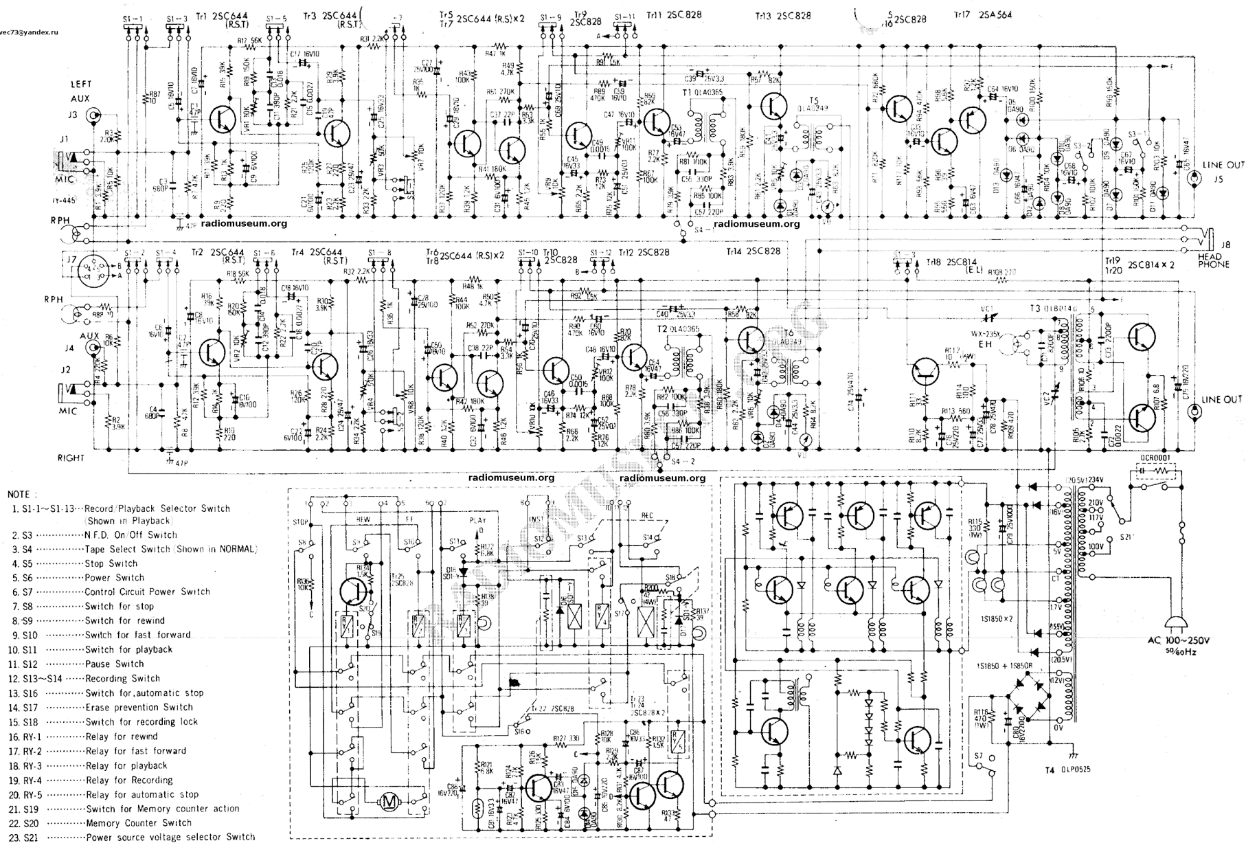
FIG. 2 — DIAGRAMA ESQUEMÁTICO ORIGINAL DO GRAVADOR MAGNETOFÔNICO "NATIONAL" RS-275US
