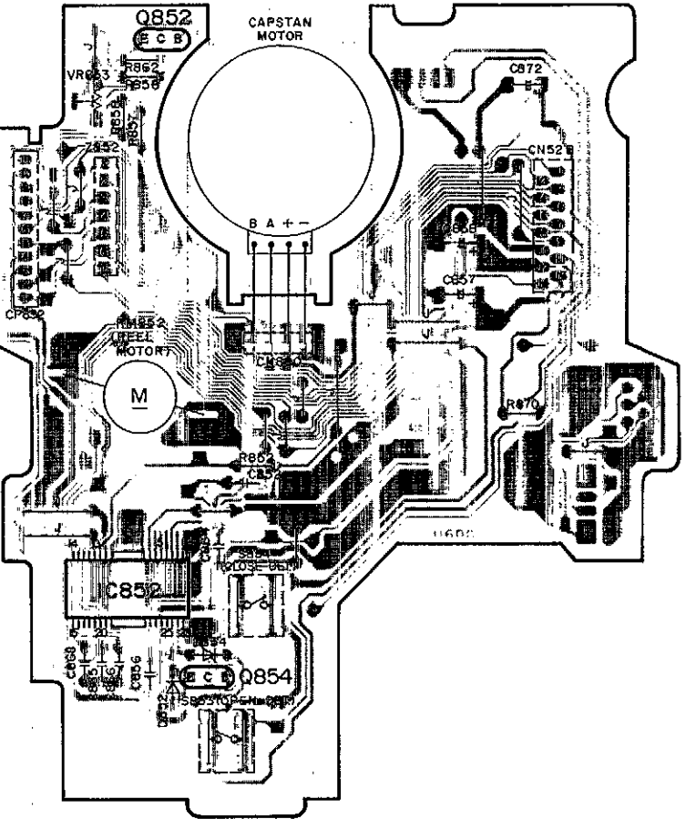
C MOTOR P.C.B.(REP1959A-T)
