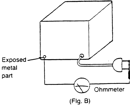
Resistance=Approx. ∞
