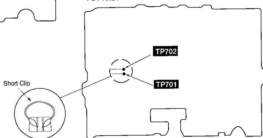
FL P.C.B.
