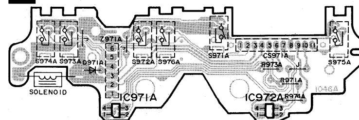
F メカニズム基板 (DECK2)
