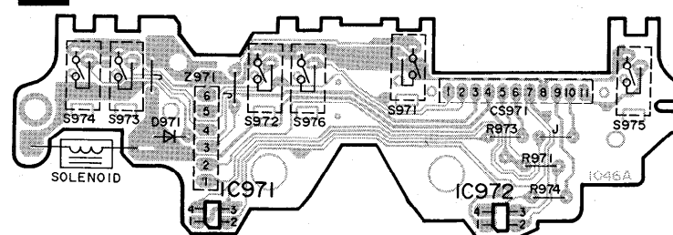
E メカニズム基板 (DECK1)
