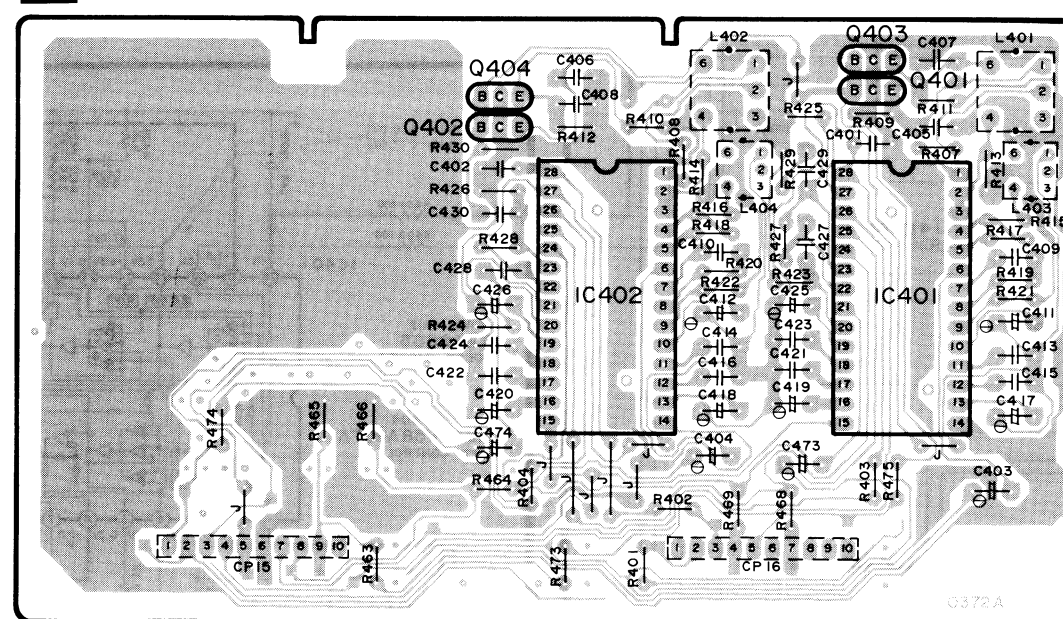
DOLBY NR P.C.B.
