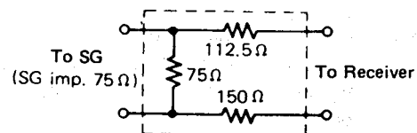
300Ω FM dummy antenna [Fig. 11] (Abb. 11)
