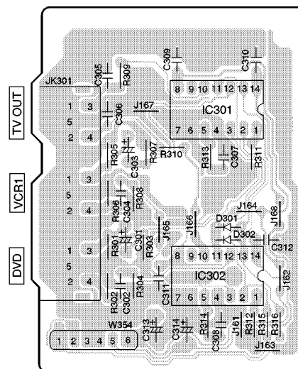
F S-VIDEO P.C.B. (REP3020E-S)
