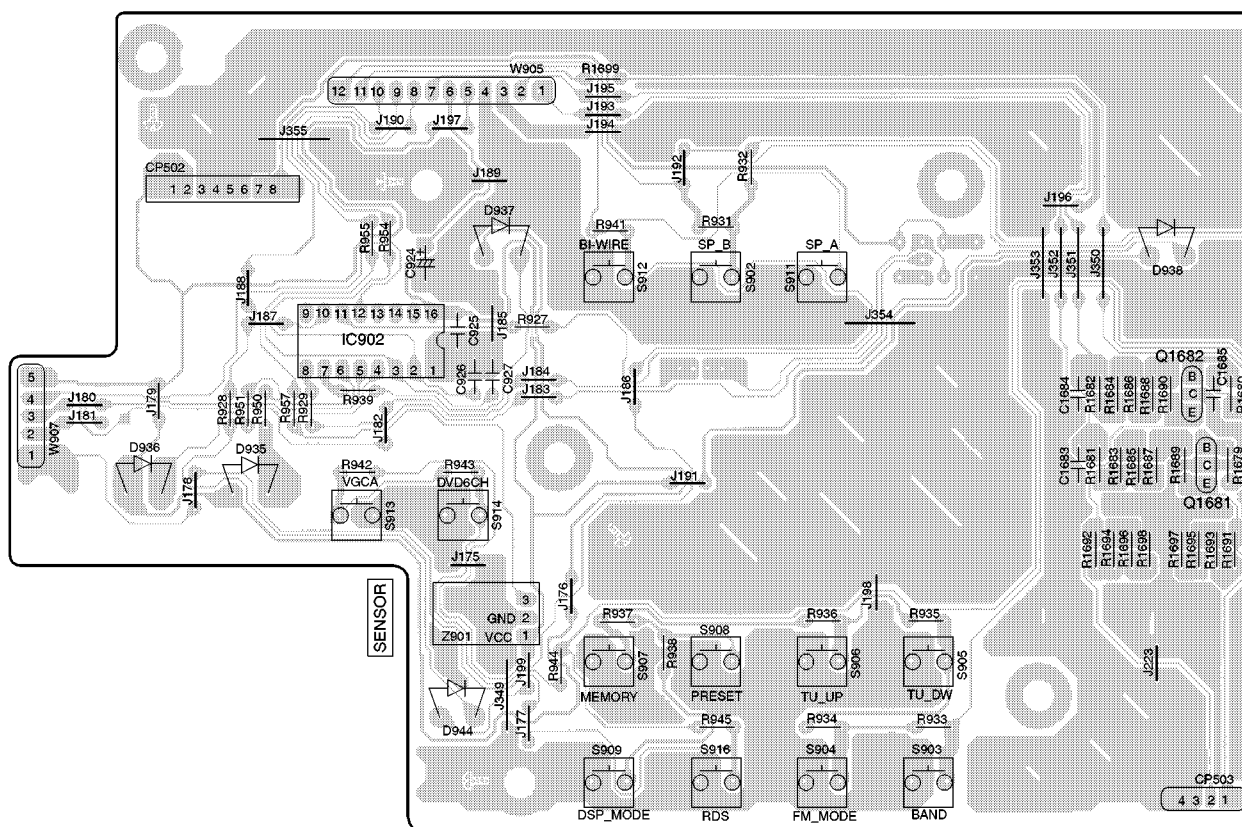
G KEY P.C.B. (REP3020E-S)
